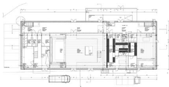
Bau einer Kulturhalle gemäss den Spezifikationen von Stoll Audio
