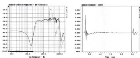
Messung der akustischen Parameter eines Beschallungssystems
